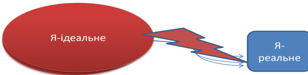
Рис. 4. Модель self-hate.
