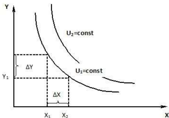
Криві байдужості
