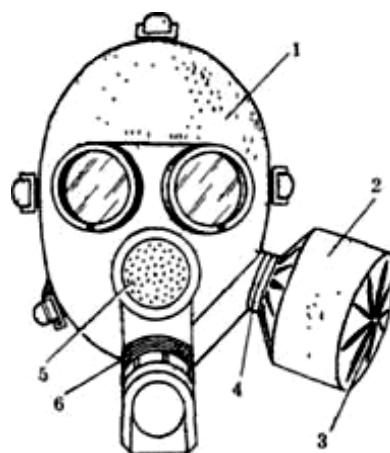
Рис. 6.10. Протигаз ЦП-7:
