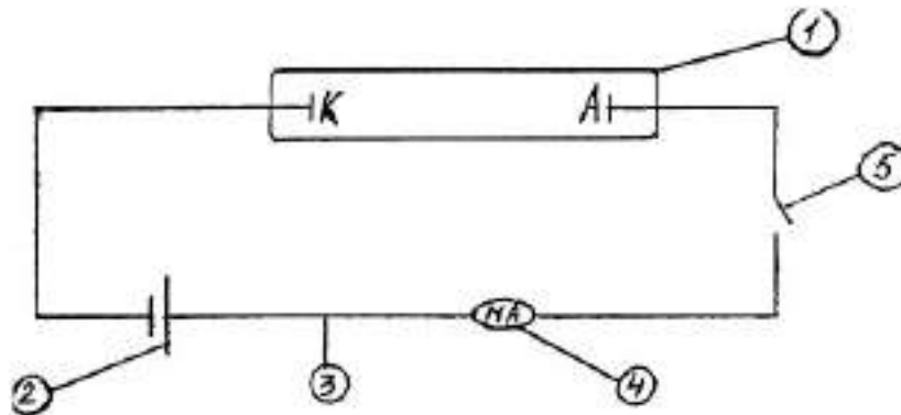
Рис. 6.3. Схема іонізаційного методу індикації:
