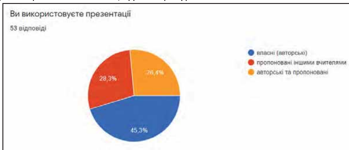
Рис. 2. Використання презентацій
