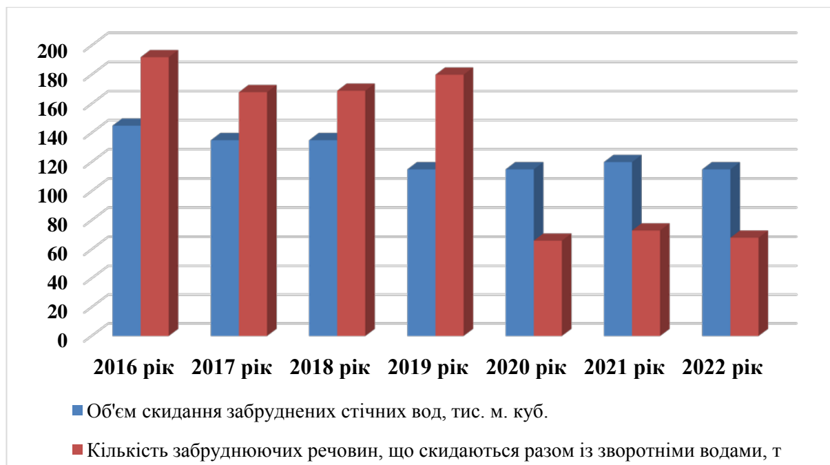
Рис. 2. Динаміка скидання забруднених стічних вод Підволочиським УЖКГ
